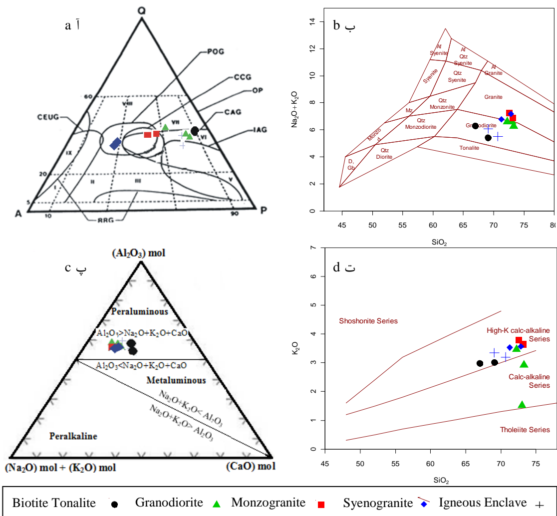
شکل ۶. ا) موقعیت نمونه‌های گرانیتوئید استند در نمودار QAP (Streckeisen, 1976) (IAG: Island Arc Granitoids, CAG: Continental Arc Granitoids, OP: Ocean Plagiogranites, CCG: Continental Collision Granitoids, POG: Post-Orogenic Granitoids, CEUG: Continental Epeigenic Uplift Granitoids, RRG: Rift-Related Granitoids), ب) موقعیت نمونه‌های گرانیتوئید استند در نمودار (Middlemost, 1994), ج) موقعیت نمونه‌های گرانیتوئید استند در نمودار (Gill, 2010) (پ) نمونه‌ها در نمودار (Middlemost, 1994), د) موقعیت نمونه‌های گرانیتوئید استند در نمودار (Peccerillo & Taylor, 1976) بیشتر در محدوده کالک‌آلکالین با پتاسیم بالا واقع شده‌اند.
