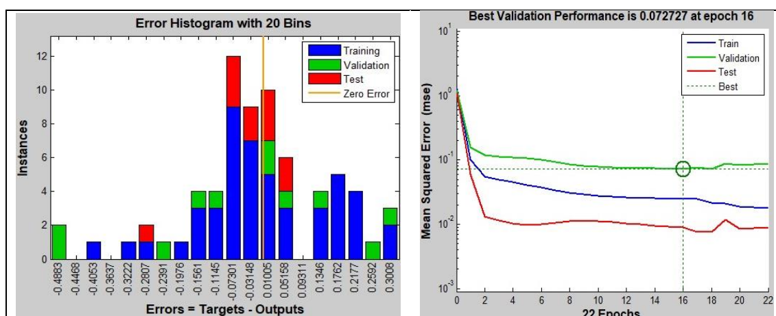
شکل ۱۶- کمترین خطای MSE (سمت راست) و هیستوگرام خطاها (سمت چپ) در مدل بهینه (در لایه مخفی ۵) Fig. 16. The lowest MSE error (right side) and histogram of errors (left side) in the optimal model (in hidden layer 5).
