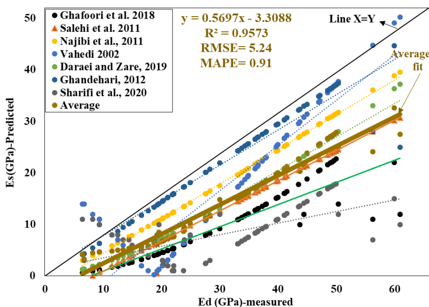
شکل ۸- مقایسه مدول الاستیسیته استاتیک حاصل از روابط روابط ارائه شده در برخی پژوهش‌ها (پژوهشگران ایرانی) بر اساس نتایج آزمایشگاهی این مطالعه با مدول الاستیسیته دینامیک اندازه‌گیری شده در این مطالعه
