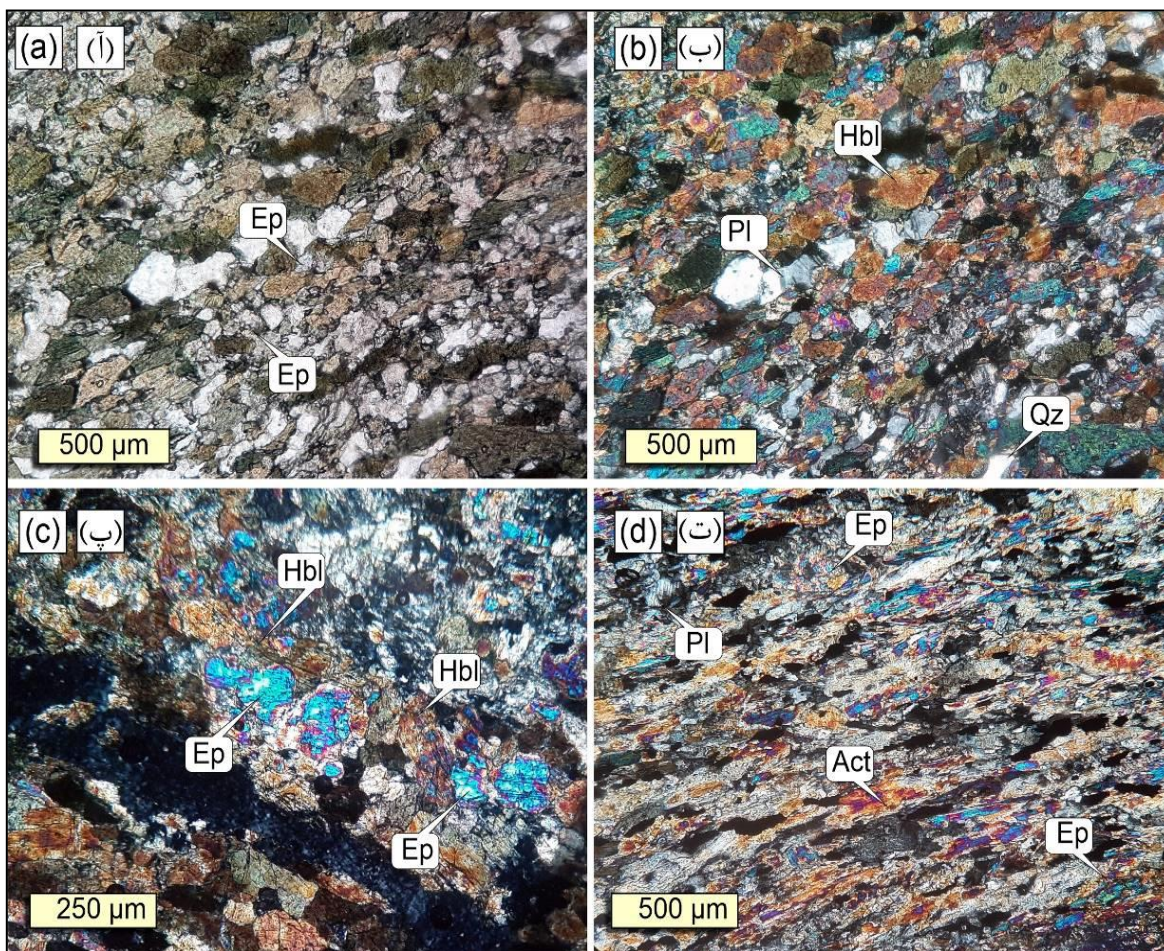
شکل ۳- تصاویر مقاطع نازک نمونه‌های مورد مطالعه. (آ) و (ب) اپیدوت آمفیبولیت با بافت گرانوبلاستیک تا نماتوبلاستیک. (پ) ناپایداری در حاشیه اپیدوت‌ها و تبدیل آنها به هورنبلند در طی افزایش درجه دگرگونی، (ت) بافت نماتوبلاستیک حاصل جهت‌گیری اکتینولیت‌های سوزنی در اکتینولیت شیسست. علائم اختصاری کانی‌ها: Act: اکتینولیت، Ep: اپیدوت، Hbl: هورنبلند، Qz: کوارتز، Pl: پلاژیوکلاز (Whitney and Evans, 2010).
