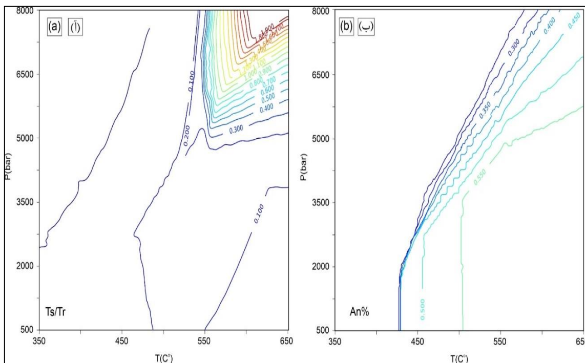
شکل ۸- خطوط هم‌ترکیب (Isopleth) محاسبه شده برای (آ) تغییرات نسبت محتوای چرماکیت به ترمولیت (Ts/Tr) در آمفیبول و (ب) آنورتیت در پلاژیوکلاز در نمودار فازی شکل ۷.
