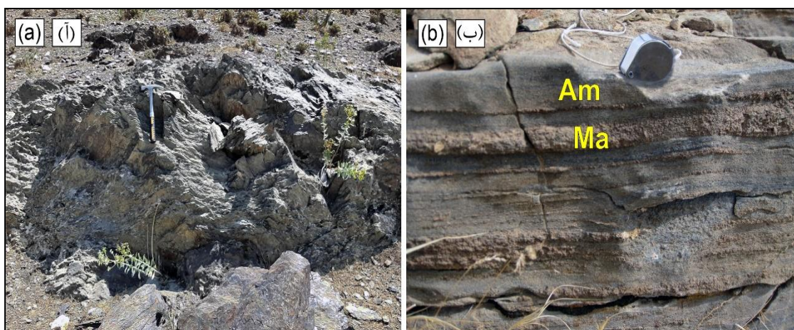
شکل ۲- (آ) بیرونزدگی‌های اکتینولیت شیست در منطقه مورد مطالعه (دید به سمت شمال غرب). برگوارگی مشخص در محل بیرونزدگی به چشم می‌خورد. (ب) توالی آمفیبولیت (Am) و مرمر (Ma).
