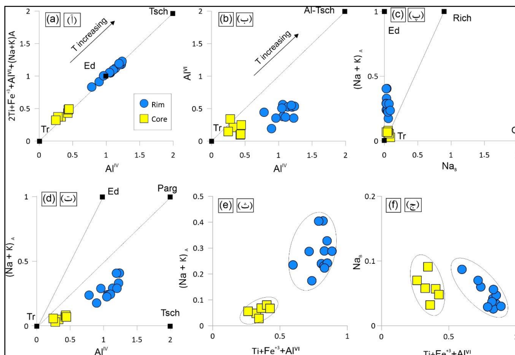
شکل ۶- جانشینی‌های کاتیونی در آمفیبول‌های مورد مطالعه. Ed: ادنیته، Parg: پارگازیت، Rich: ریشتریت، Tsch: چرماکیت.
