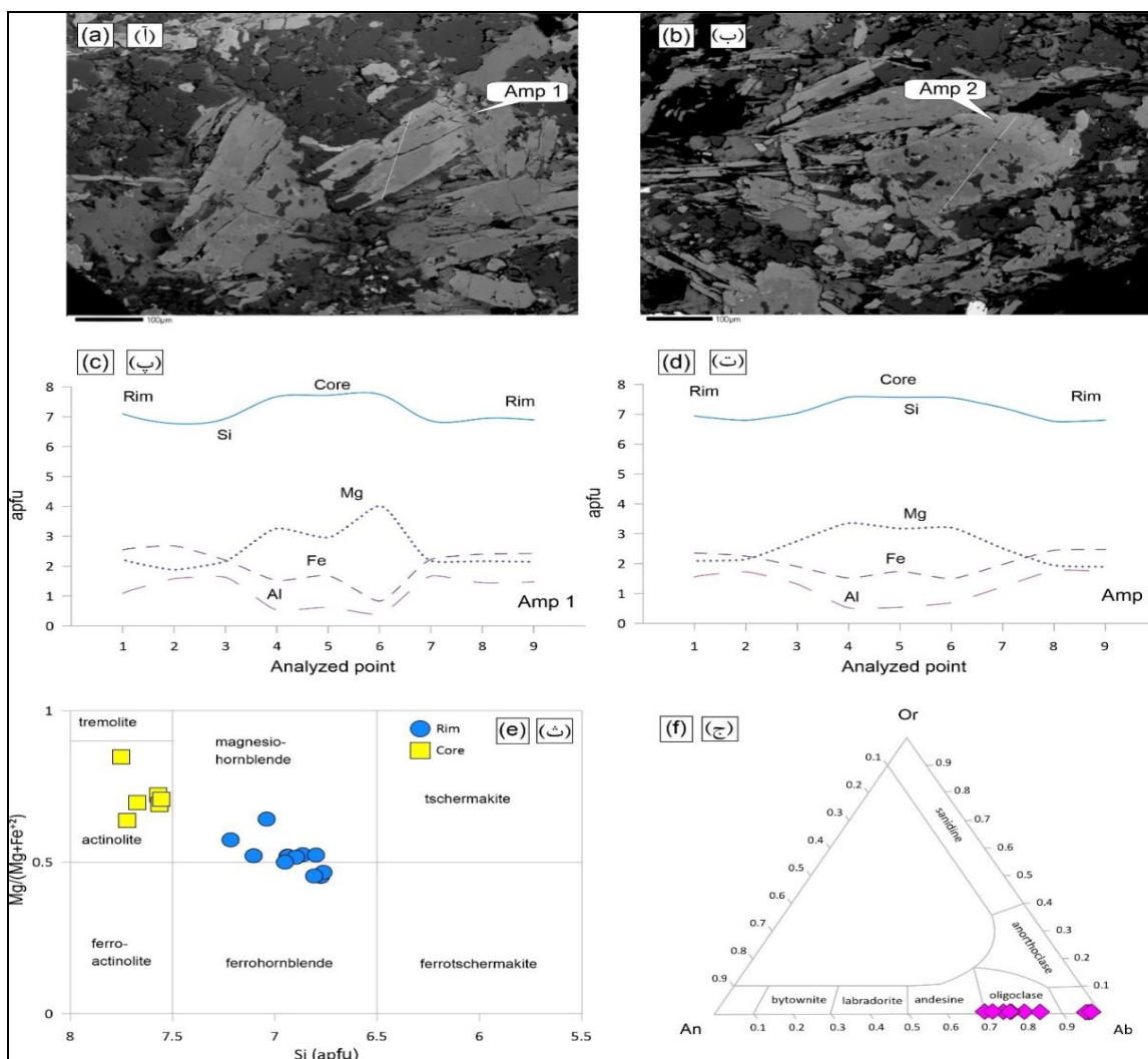
۴- (ا) و (ب) تصاویر میکروسکوپ الکترونی از نمونه‌های مورد مطالعه که مسیرهای پروفیل‌های شیمیایی تهیه شده از آمفیبول‌ها (خطوط سفید رنگ) را نشان می‌دهند؛ (پ) و (ت) تغییرات شیمیایی عناصر Si، Mg، Al و Fe در آمفیبول‌های تجزیه شیمیایی شده؛ (ث) نمودار رده‌بندی آمفیبول‌های کلسیک (Hawthorn and Oberti, 2007)؛ (ج) نمودار رده‌بندی شیمیایی فلدسپارها برای پلاژیوکلازهای مورد مطالعه (Deer et al., 1963).
