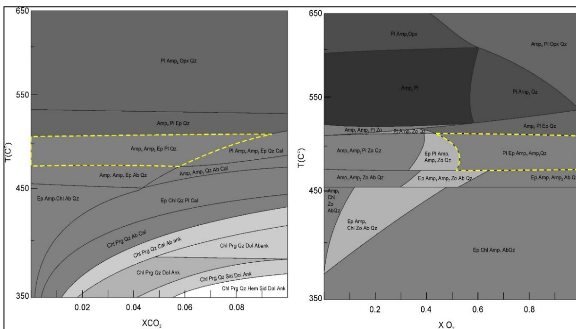
شکل ۹- (ا) نمودار فازی T-XCO_2 و (ب) نمودار فازی T-XO_2 محاسبه شده با استفاده از ترکیب شیمیایی نمونه EA01. علائم اختصاری کانی‌ها مشابه با شکل ۷. خط چین‌ها مرز مجموعه‌های پایدار در نمونه‌های مورد مطالعه با سایر مجموعه‌ها را نشان می‌دهند.
