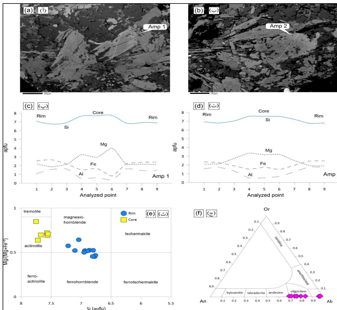
۴- (آ) و (ب) تصاویر میکروسکوپ الکترونی از نمونه‌های مورد مطالعه که مسیرهای پروفیل‌های شیمیایی تهیه شده از آمفیبول‌ها (خطوط سفید رنگ) را نشان می‌دهند؛ (پ) و (ت) تغییرات شیمیایی عناصر Si، Mg، Al و Fe در آمفیبول‌های تجزیه شیمیایی شده؛ (ث) نمودار رده‌بندی آمفیبول‌های کلسیک (Hawthorn and Oberti, 2007)؛ (ج) نمودار رده‌بندی شیمیایی فلدسپارها برای پلاژیوکلازهای مورد مطالعه (Deer et al., 1963).
