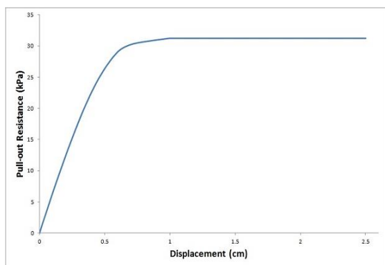
شکل ۱۹- تغییرات مقاومت در برابر تغییرمکان میخ B4 Fig. 19. Changes in strength to nail displacement B4
