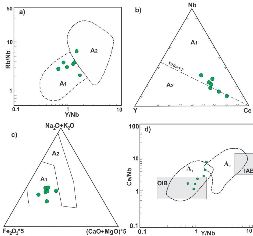
شکل ۱۰- نمودار متمایزکننده گرانیت‌های A1 و A2. نمودار نسبت Rb/Nb در برابر نسبت Y/Nb (Eby, 1992). نمودار سه تایی Y-Nb-Ce (Eby, 1992). نمودار سه تایی (CaO+MgO)*5-(Na_2O+K_2O)-Fe_2O_3*5 (Grebennikov, 2014). نمودار نسبت Ce/Nb در برابر نسبت Y/Nb (Eby, 1992).
