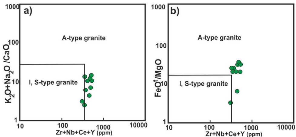
شکل ۸- نمودارهای متمایز کننده گرانیت‌های نوع A از گرانیت‌های نوع I و S (Whalen et al., 1987). نمودار (a) Zr+Ce+Y+Nb در برابر نسبت (Na_2O+K_2O)/CaO . نمودار (b) Zr+Ce+Y+Nb در برابر نسبت FeO^t/MgO . A-type= Anorogenic type, I and S type= Igneous and Sedimentary types
