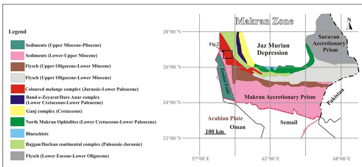
شکل ۱- نقشه ساده شده‌ای از واحدهای سنگی و ساختاری منشور برافزایشی مکران، جنوب ایران (McCall, 2002).
