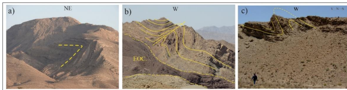
شکل ۳- a) چین برگشته با جهت میل به سمت جنوب شرق در توالی‌های ائوسن، بخش داخلی قوس ساختاری بیرجند (خط A در شکل ۲). b) چین در واحدهای شیل و ماسه‌سنگ قرمز ائوسن. c) چین برگشته در شیل منطقه چاه‌حوض با میل به سمت جنوب.
