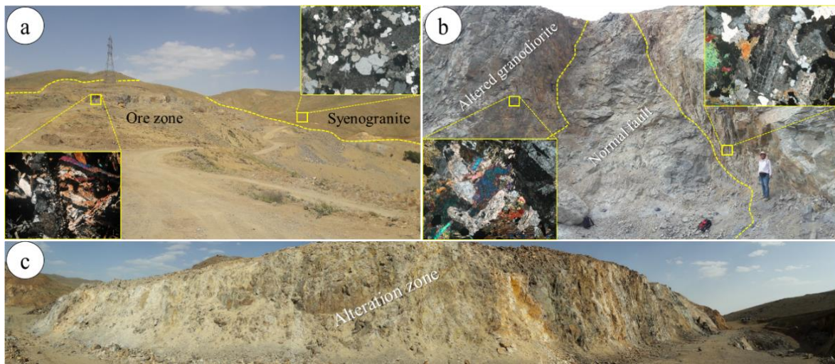
شکل ۳- a) تصاویر صحرایی از موقعیت قرارگیری گرانیتوئید دگرسان شده و میزبان کانه‌زایی نسبت به پهنه معدنی، در بخش شمال غربی کانسار چوره‌ناب. b) رخنمون واحد گرانودیوریت تکتونیزه و به شدت دگرسان شده. c) نمای کلی از پهنه دگرسانی کانسار چوره‌ناب. دید تصویر به سمت شمال محدوده مورد مطالعه است.
