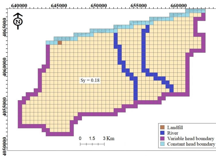
شکل ۱۱- مقدار آبدهی ویژه واسنجی شده مدل دشت بابلسر Fig.11. The calibrated specific yield of the case study
