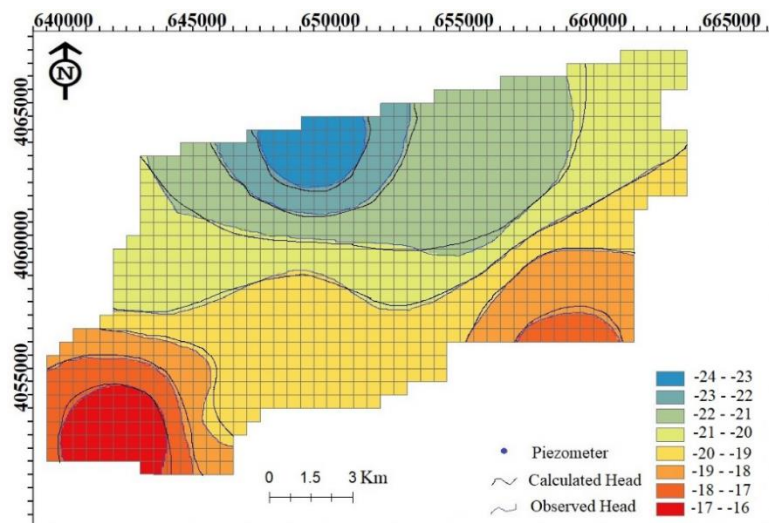
شکل ۱۰- بار آبی مشاهداتی و شبیه‌سازی شده مدل در پایان واسنجی در شرایط ناپایدار (اسفند ۱۳۹۱) Fig.10. The observation and calculation head at the end of the calibration period in unsteady state (March 2012)
