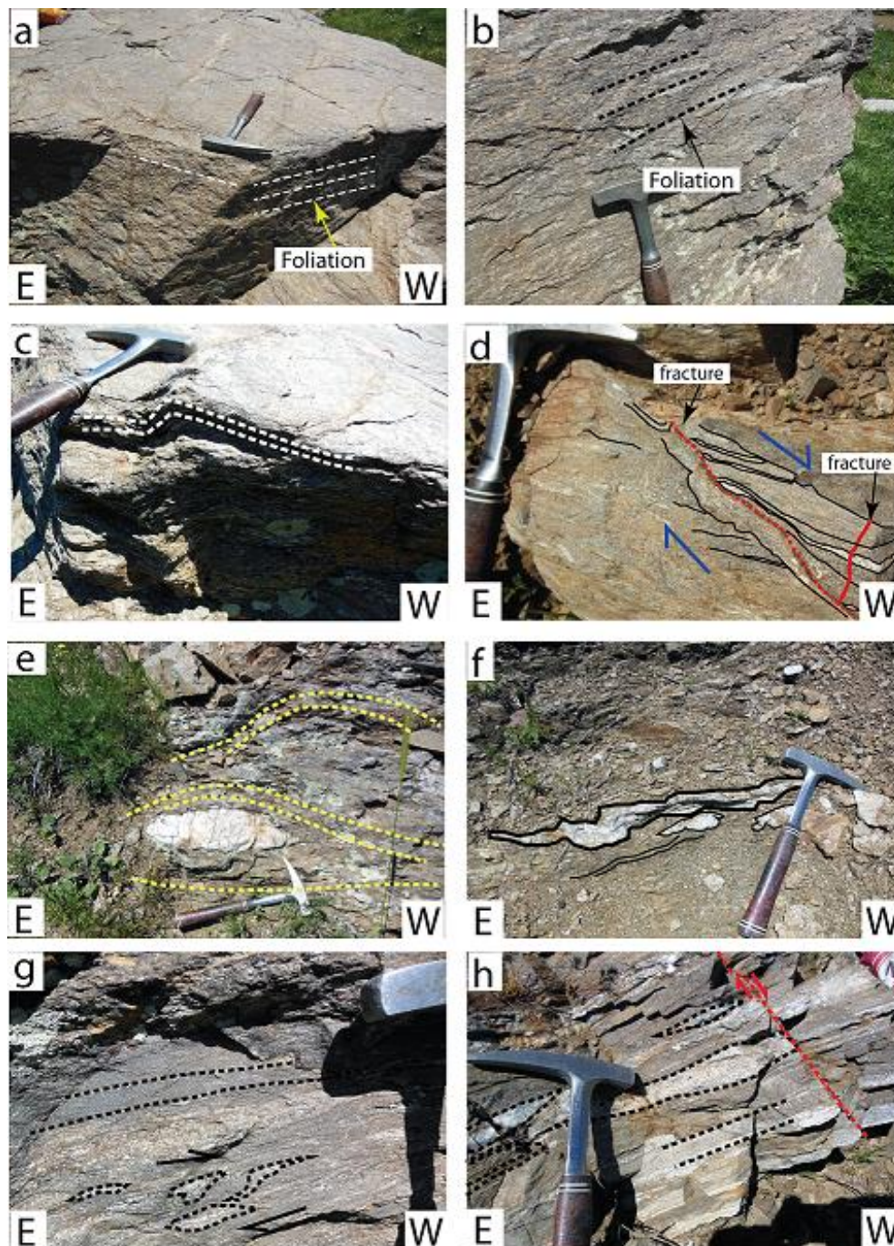
شکل ۳- تصاویر صحرایی از میکاشیست‌های غرب سیلوانا. (a و b) برگواگی در میکاشیست‌ها. (c) ساختار کینک‌باند. (d) تأثیر نیروهای برشی راست‌گرد بروی میکاشیست‌ها. (e) ساختار بودیناژ در رگه‌های سیلیسی. (f) رگه‌های سیلیسی با دگرشکلی نامتقارن. در برخی موارد ساختارهای سیگموئیدی در رگه‌ها تشکیل شده است. (g) ساختارهای سیگموئیدی. (h) لایه‌بندی و ساختارهای سیگموئیدی.
