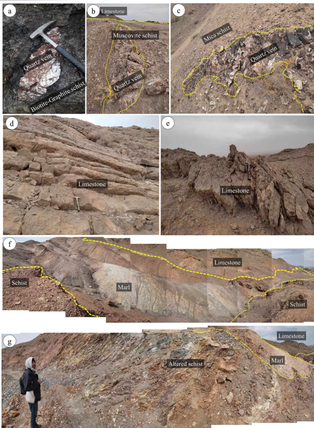
شکل ۴- a، b و c) تشکیل عدسی‌ها و رگچه‌های کوارتزی در داخل سنگ‌های دگرگونی؛ d و e) رخمون سنگ‌آهک‌های بلورین مربوط به مجموعه دگرگونی کوه‌دم در بخش غربی محدوده بندچرک؛ f) همبری شیست حاوی گرافیت با مارن و سنگ‌آهک، و g: واحدهای شیستی دگرسان‌شده در بخش زیرین واحدهای مارنی.
