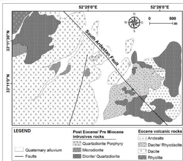
شکل ۲- نقشه زمین‌شناسی ساده شده منطقه اکتشافی ظفرقند. پس از تغییرات از اعلمی‌نیا و همکاران (Alaminia et al., 2017). Fig. 2. Simplified geological map of the Zafarghand exploration area (adapted from Alaminia et al., 2017).
