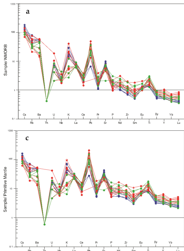
شکل ۸-۱. (a, b) عادی سازی عناصر نادر خاکی (REEs) و عناصر فرعی نمونه‌ها به N-MORB (مورب نرمال) و E-MORB (مورب غنی شده) (Boynton, 1984; Sun and McDonough, 1989) عادی سازی عناصر نادر خاکی (REEs) و عناصر فرعی نمونه‌ها به (گوشته اولیه) و Chondrite (کندریت). (c, d) عادی سازی عناصر نادر خاکی (REEs) و عناصر فرعی نمونه‌ها به primitive mantle (مورب غنی شده) و chondrite (کندریت) (Boynton, 1984; Sun and McDonough, 1989).
