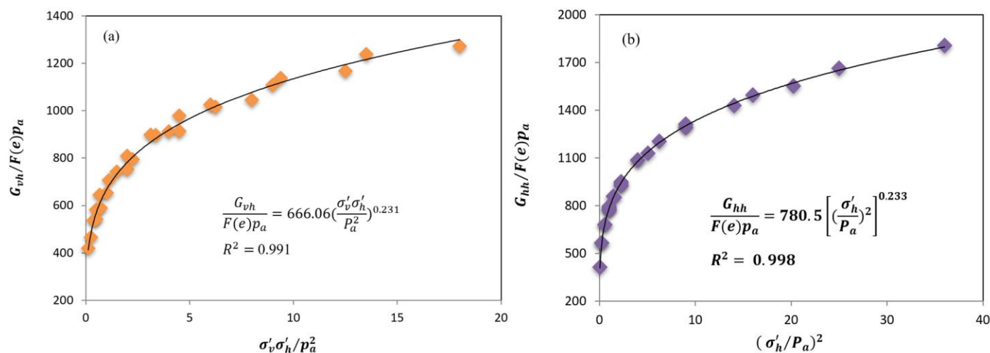
شکل ۳- فرایند محاسبه مولفه‌های ناهمسانی ساختار بافتی خاک در ماسه تسینو: (a) برازش منحنی بر روی زوج داده \left( \frac{G_{vh}}{F(e)p_a} - \frac{\sigma'_v \sigma'_h}{p_a^2} \right) برای بدست آوردن A_{vh} (b) برازش منحنی بر روی زوج داده \left( \frac{G_{hh}}{F(e)p_a} - \left( \frac{\sigma'_h}{p_a} \right)^2 \right) جهت محاسبه A_{hh}
