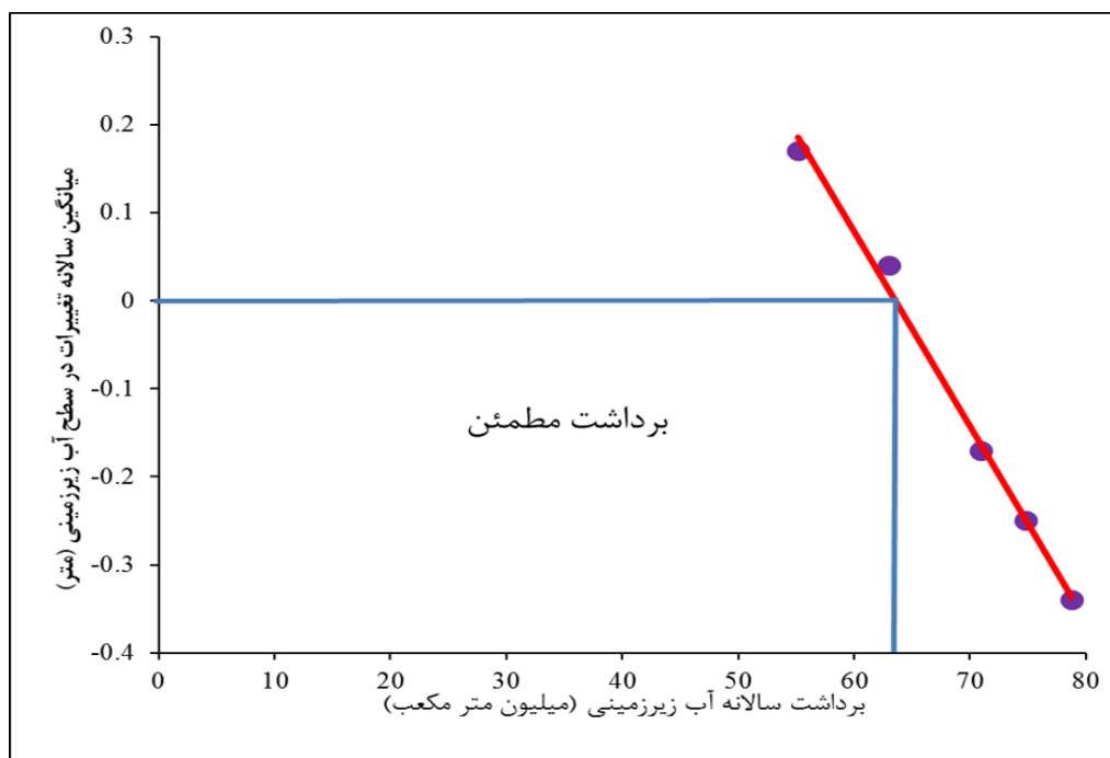
شکل ۴- تعیین برداشت مطمئن در آبخوان داورزن.
