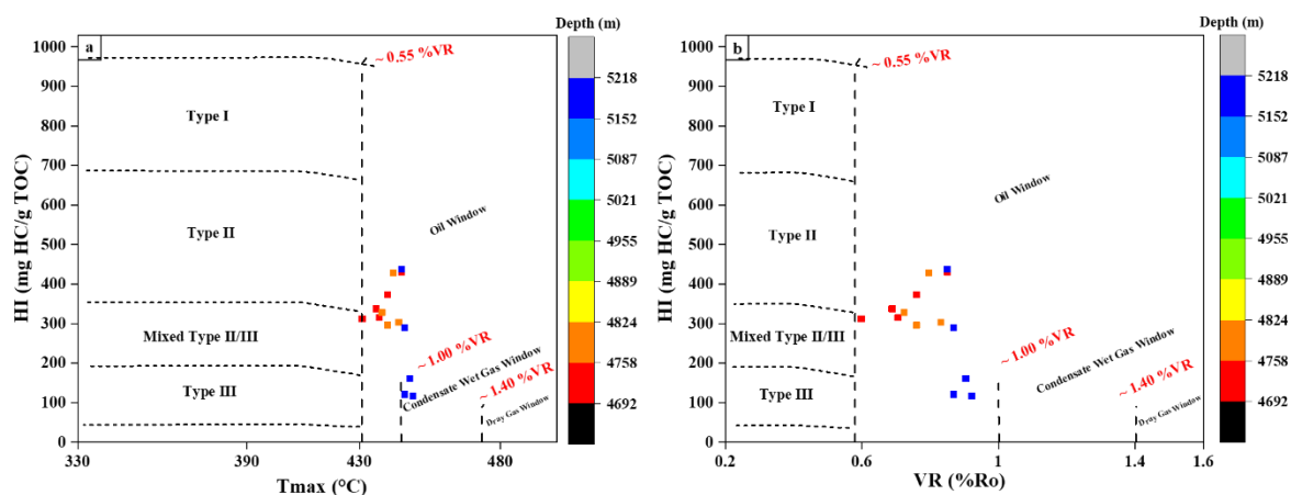
شکل ۷- (a) نمودار HI در مقابل Tmax؛ (b) نمودار HI در مقابل انعکاس ویتترینیت نمونه‌های مورد مطالعه (اقتباس از Abeer et al., 2011) Fig. 7. a) Plot of HI against Tmax; b) HI vs. VR diagram of studied samples (adopted from Abeer et al., 2011)
