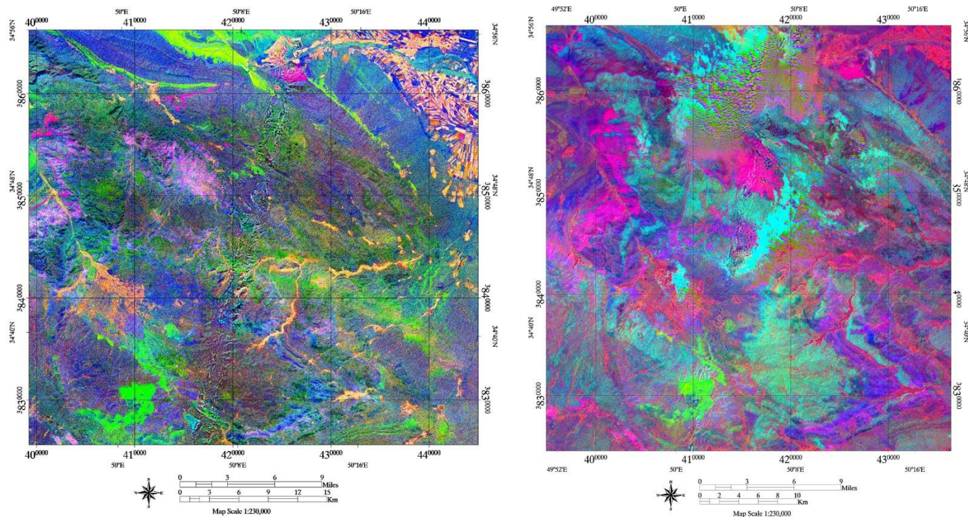
شکل ۱۴- نتیجه پردازش به روش آنالیز مولفه اصلی-انتخابی (تصویر سمت چپ) و پردازش به روش نسبت باندی (تصویر سمت راست) Fig. 14. Result of processing using the Principal Component Analysis-Selective method (left image) and processing using the Band Ratio method (right image)
