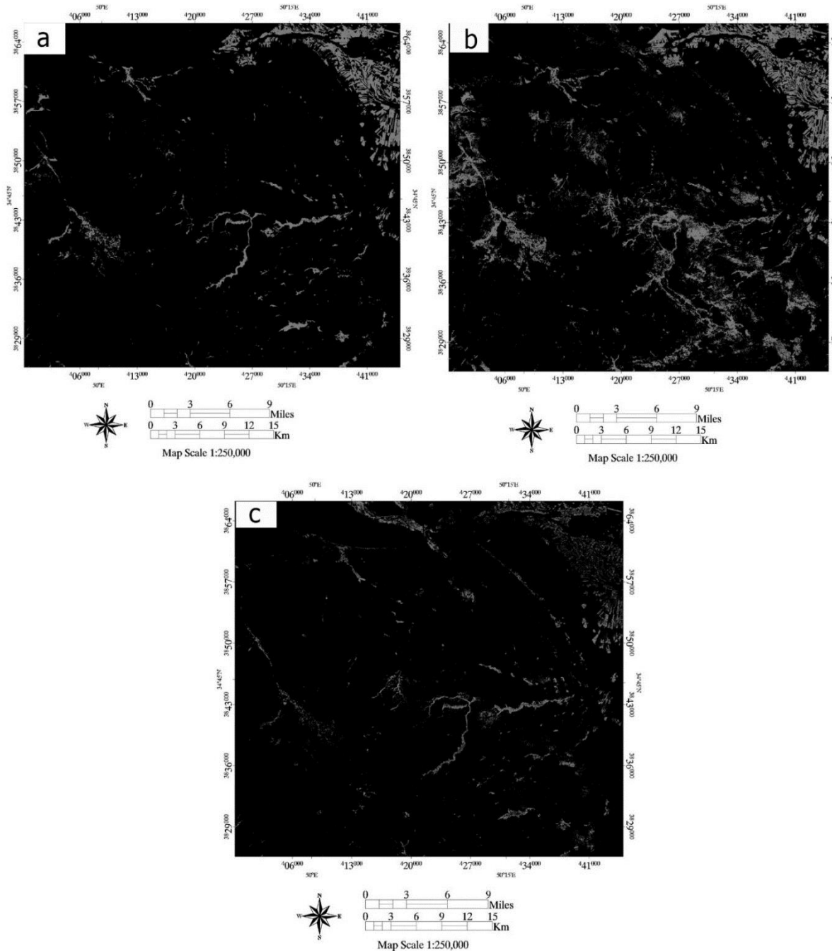
شکل ۱۷- (a) بارسازی دگرسانی آرژیلیک، (b) پروپلیتیک و (c) فیلیک به روش نقشه بردار زاویه طیفی Fig. 17. Highlighting (a) argillic, (b) propylitic, and (c) phyllic alteration using the spectral angle vector mapping method.
