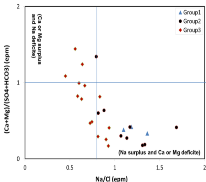
شکل ۱۳- رابطه بین \text{Ca}+\text{Mg}/\text{SO}_4+\text{HCO}_3 در مقابل نسبت \text{Na}/\text{Cl} در نمونه‌های آب‌های زیرزمینی دشت سبزوار
