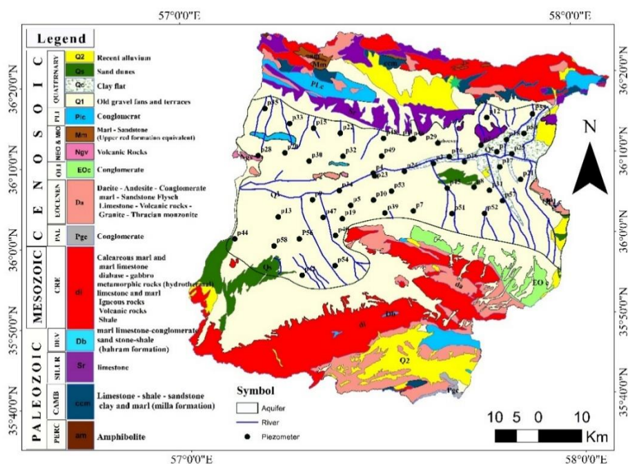
شکل ۱- نقشه زمین‌شناسی و موقعیت پیزومترهای آبخوان سبزوار
