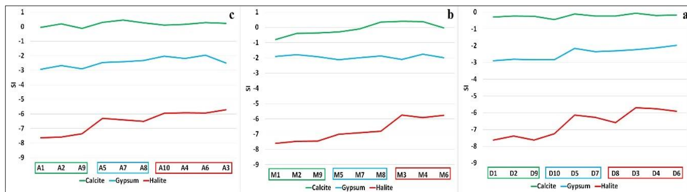
شکل ۱۱- شاخص اشباع کانی‌های کلسیت، ژئوپس و هالیت دوره‌های (a) دی ماه ۱۳۹۶، (b) مرداد ماه ۱۳۹۷ و (c) آبان ماه ۱۳۹۷ Fig. 11. Saturation index of calcite, gypsum, and halite minerals for the periods of a) January 2018, b) August 2018 and c) November 2018
