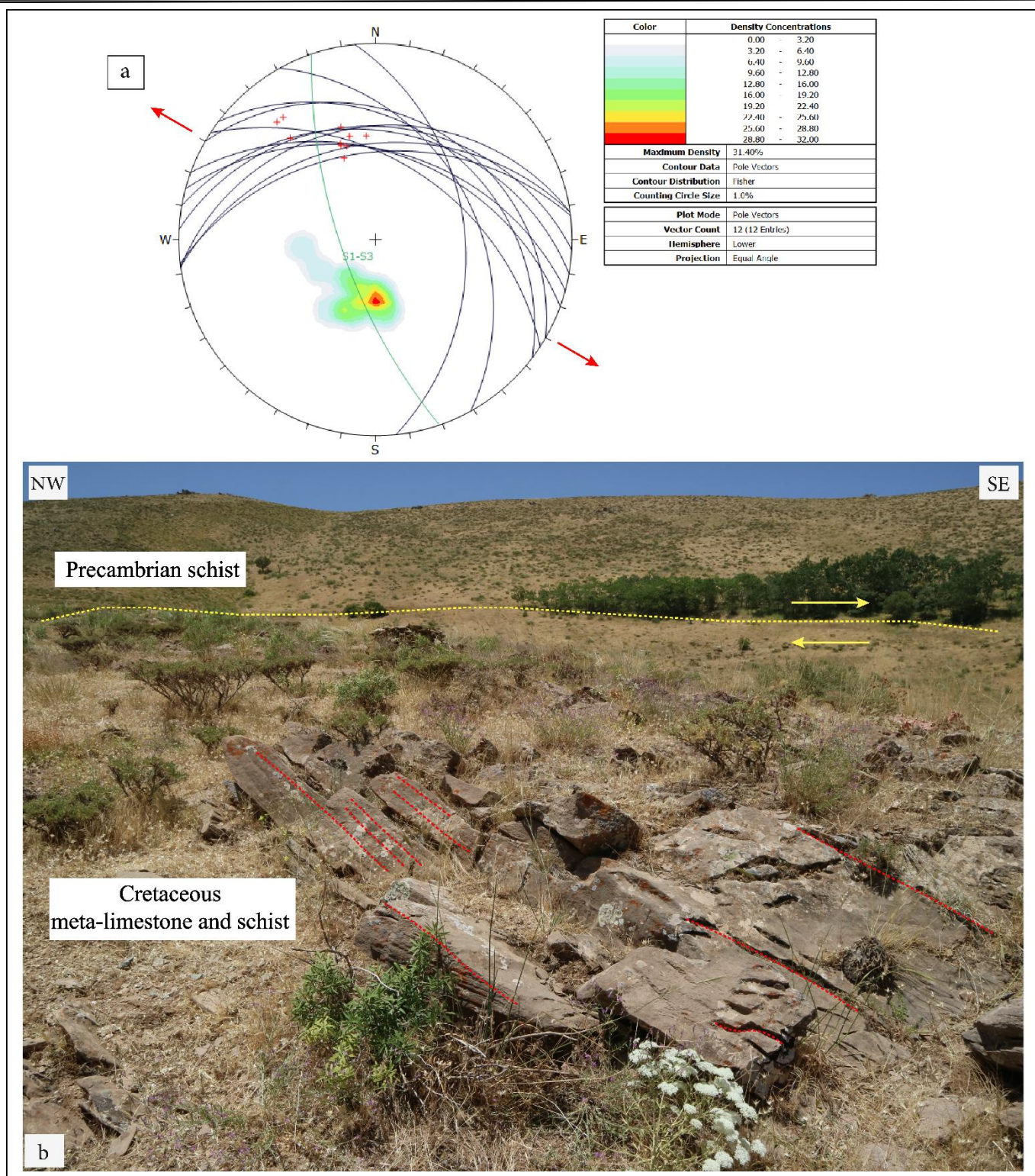
شکل ۶- (a) تصویر نیمکره پایینی شبکه اشمیت از مجموع داده‌های برداشت شده در ایستگاه ۳، شامل صفحات برگوارگی ایجاد شده در رخمون دگرگونی شیستی (کمان‌های بزرگ مشکی)، خطوارگی‌های ناشی از کشیدگی روی شیستوزیتی (بعلاوه‌های قرمز) و قطب برگوارگی‌ها. نقاط قرمز تصویر خطوارگی است و تمرکز
