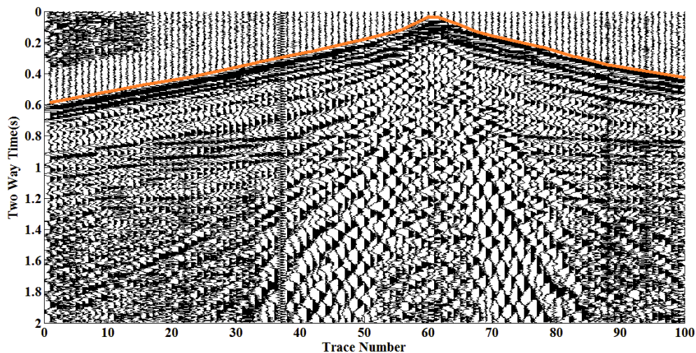
شکل ۱۰- انتخاب زمان اولین رسیده‌ها با اعمال الگوریتم نسبت انرژی روی قسمتی از برداشت چشمه مشترک.
